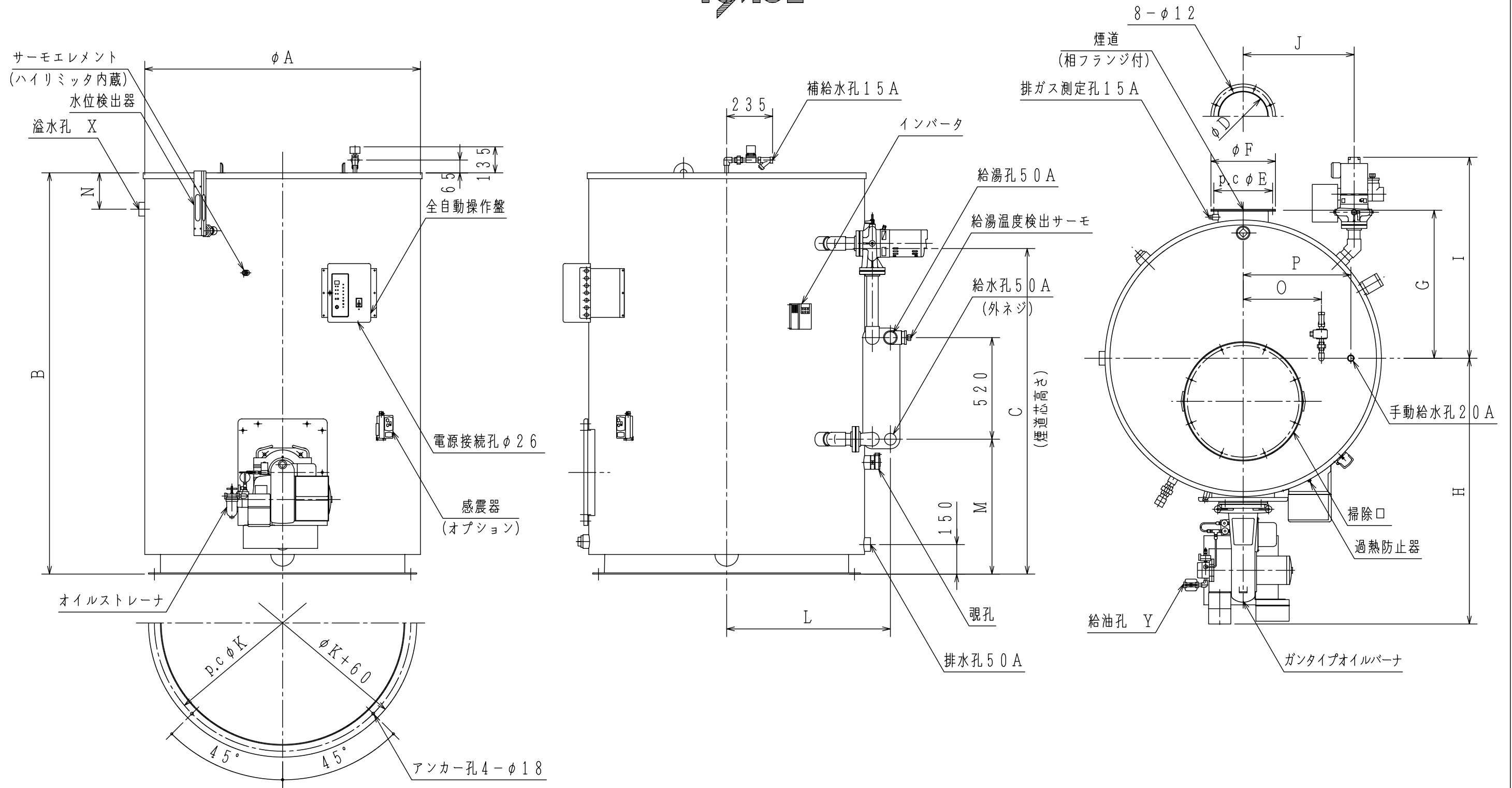
寸法表
